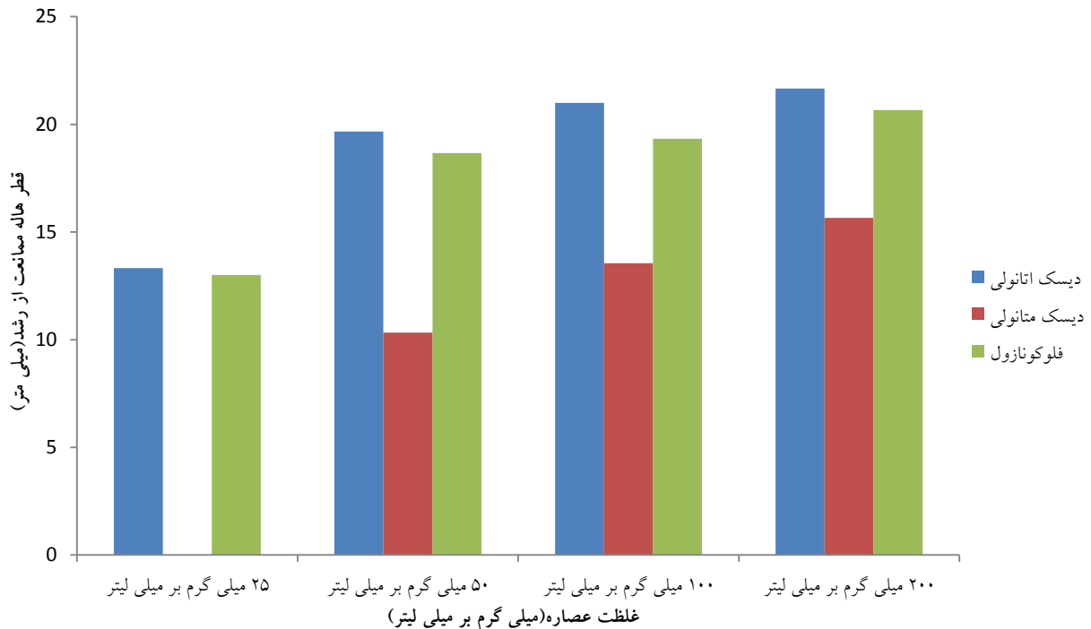
نمودار ۱: مقایسه اثر مهارکنندگی عصاره اتانولی، متانولی با فلوکونازول بر کاندیدا آلیکنس (NCPF 3153)
